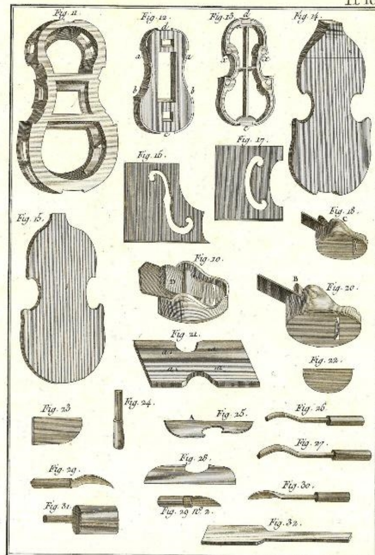
Luthier, outils propres à la facture des Instruments à Archet. 73
